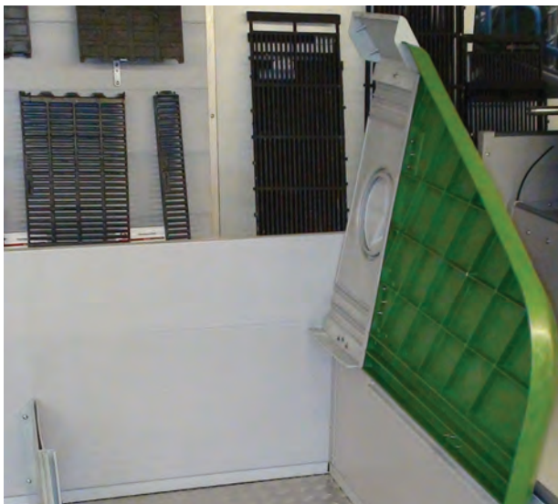
Уголок с горизонтальной клеткой опороса
