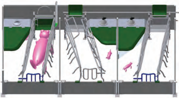
Уголок с диагональной клеткой опороса
